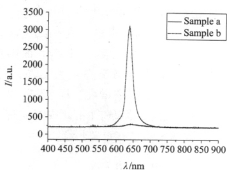
图3 样品 a,b 的端面发射光谱( I_{\text{pump}} = 1.011 \text{ mJ/cm}^2 )
