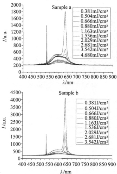
图6 YAG 激光泵浦垂直表面发射光谱
