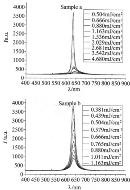
图5 YAG 激光泵浦端面发射光谱
