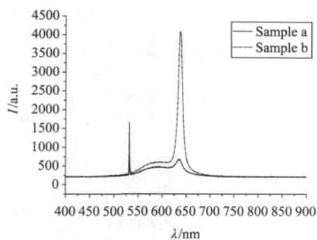
图4 样品 a,b 的垂直表面发射光谱( I_{\text{pump}} = 3.542 \text{ mJ/cm}^2 )
