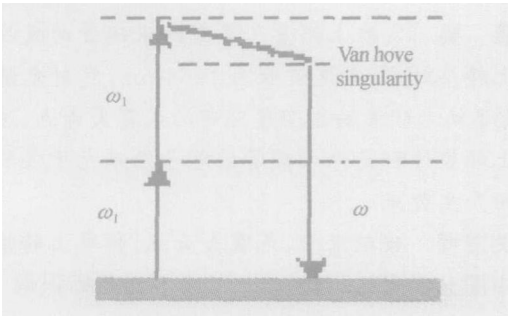
图 3 多壁碳纳米管的频率上转换产生的过程 Fig. 3 The optical frequency upconversion process of M WNTs
